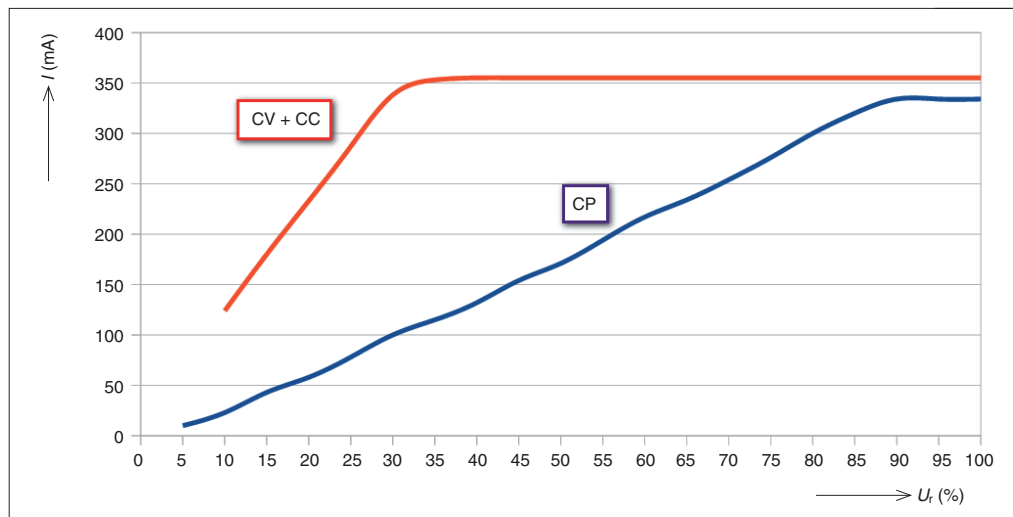
Obr. 2. Porovnání průběhu výstupního proudu napájecích zdrojů CP a CV+CC při stmívání
