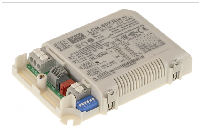
Obr. 1. Nový typ zdroje LCM s KNX vstupem
