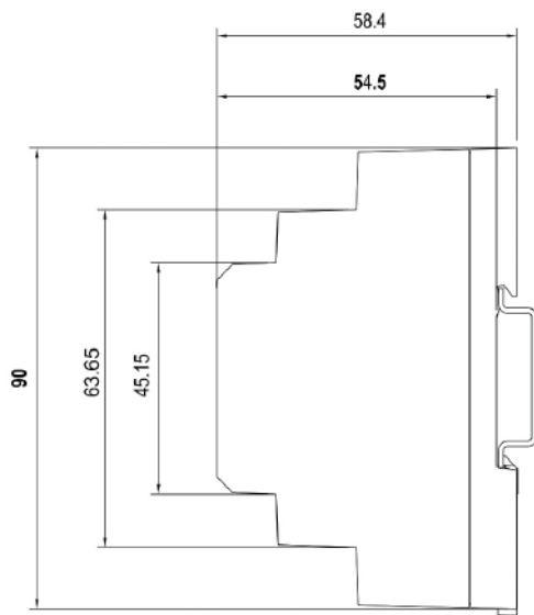
Jističový profil zdroje HDR
