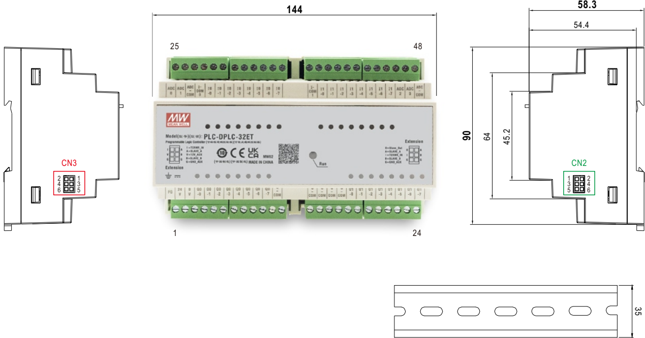
ADMISSIBLE DIN-RAIL:TS35/7.5 OR TS35/15
